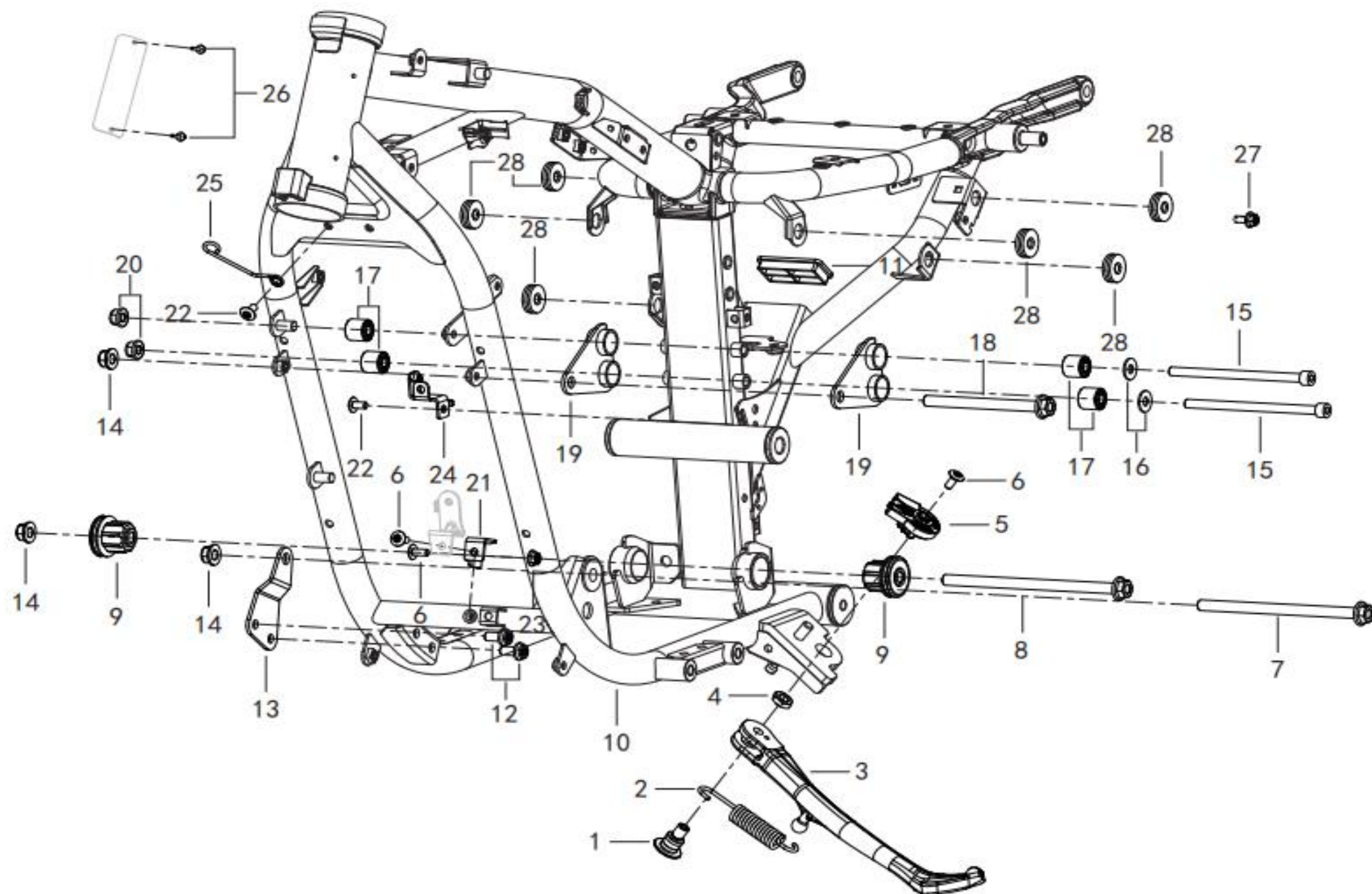
F10 车架总成 FRAME BODY ASSY.
