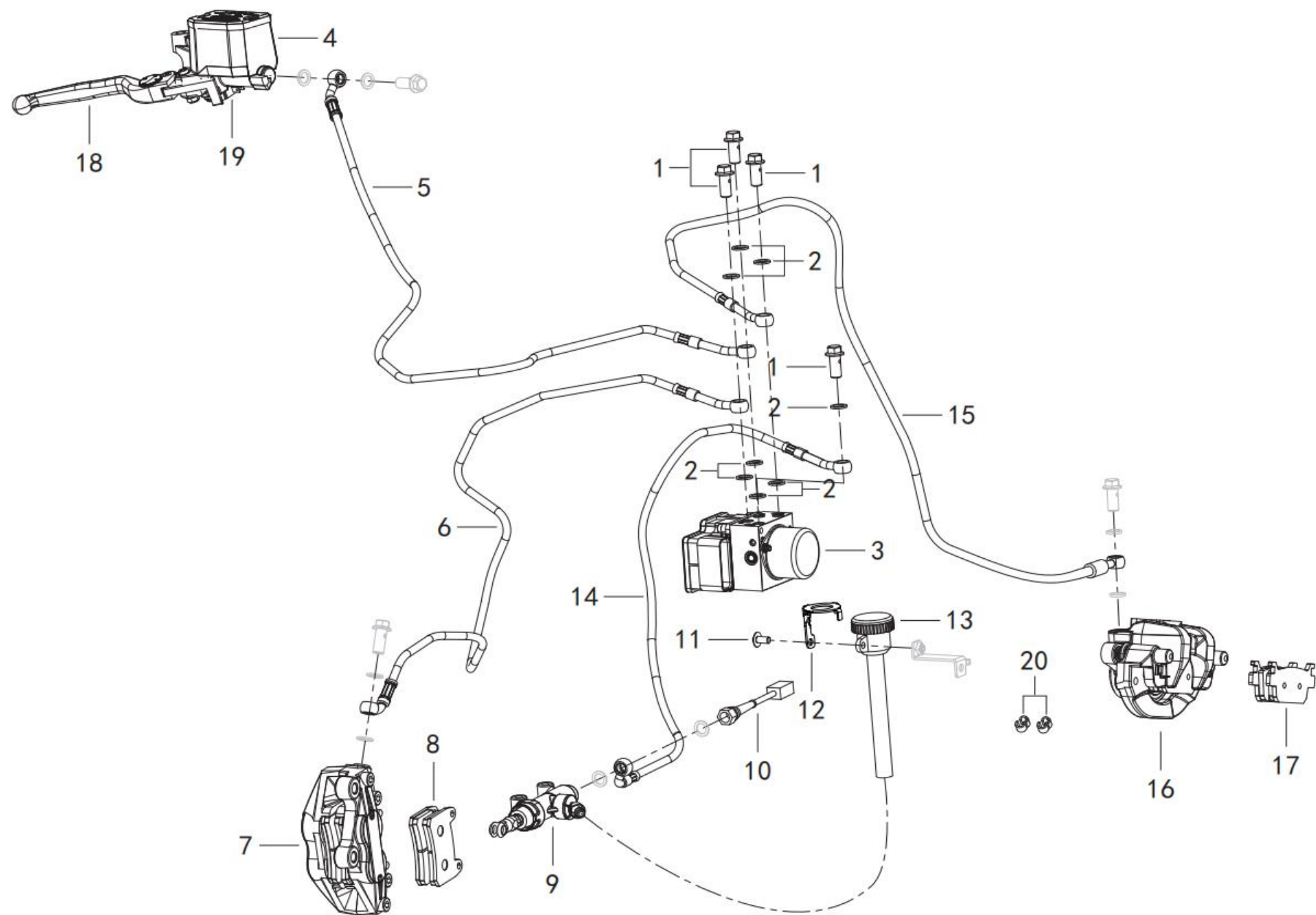
F04 液刹总成 BRAKE ASSY.
